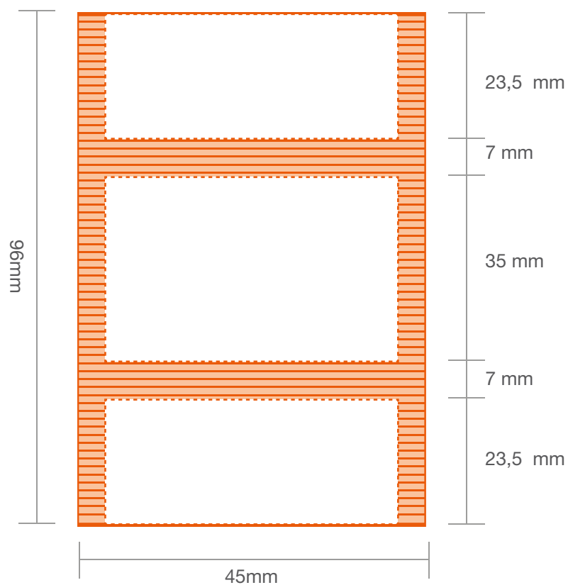
Fig. 3: Plano
